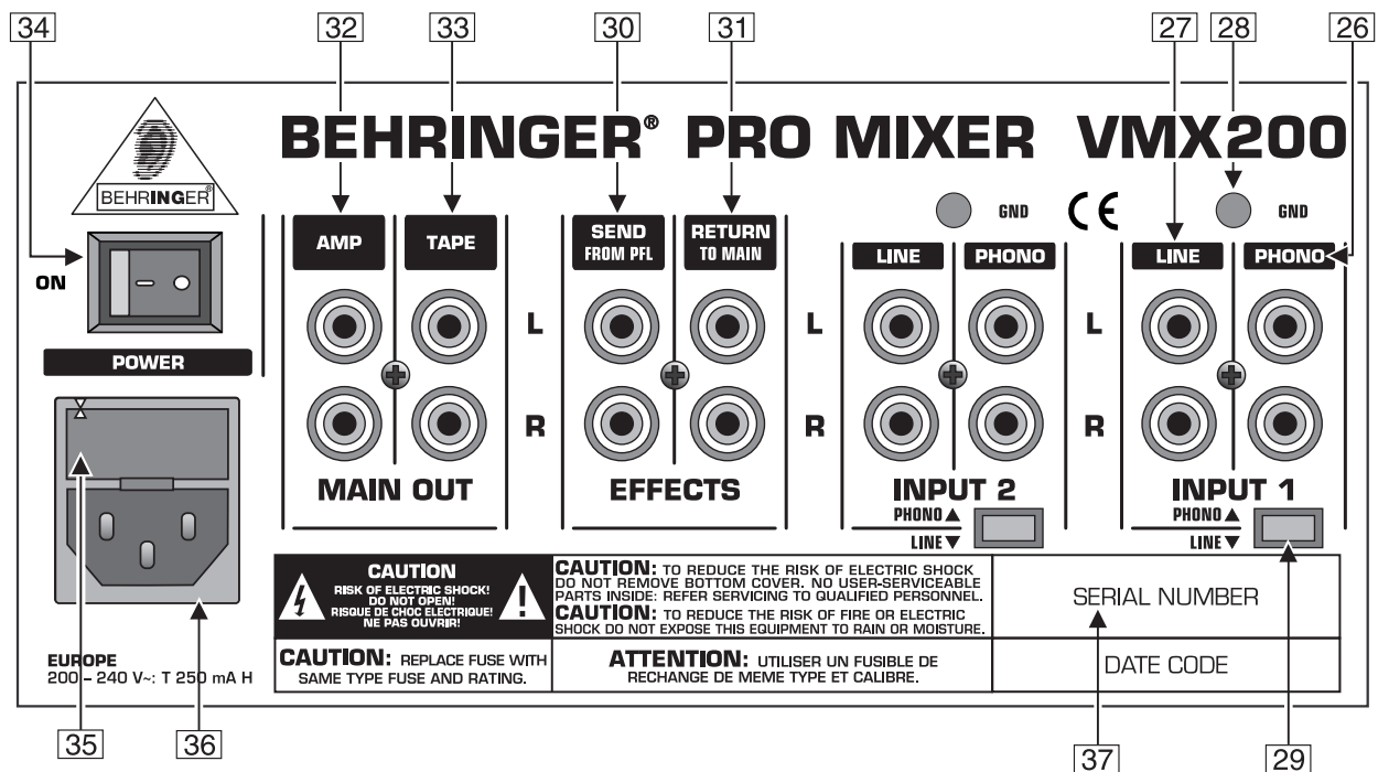
Abb. 3.1: Rückseite des VMX200
