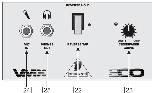
Abb. 2.1: Bedienungselemente des PRO MIXER VMX200
